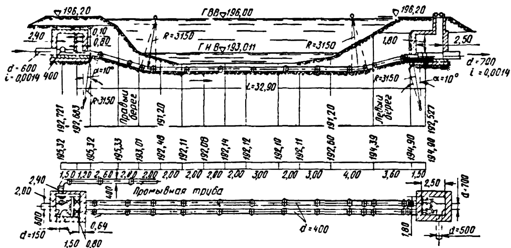
Рис. 3. Схема дюкера
